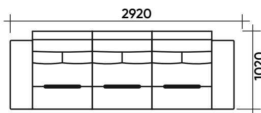
Диван А1Л-А1С-А1П
